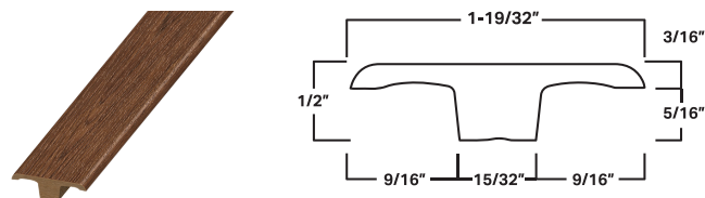
T-molding
