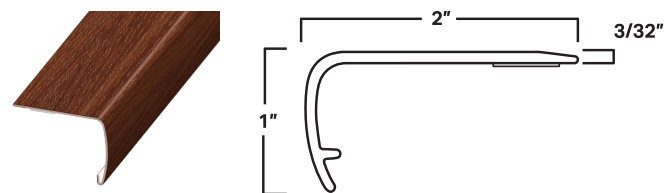
Stairnose
