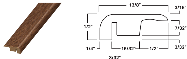
End Cap
